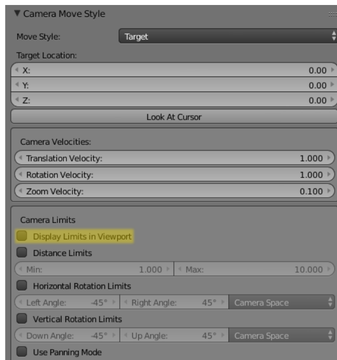
Fig. 14.2: Настройки ограничения движения камеры
