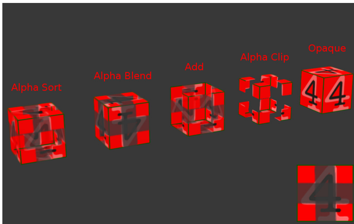
Fig. 15.2: Движком поддерживаются все типы прозрачности, доступные в Blender.
