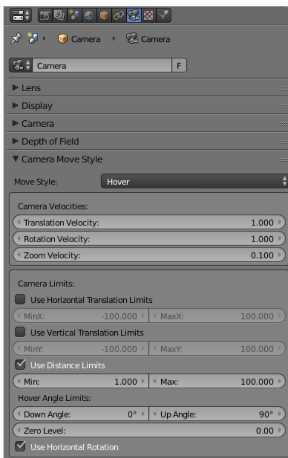
Fig. 14.1: Настройки, доступные для камеры
